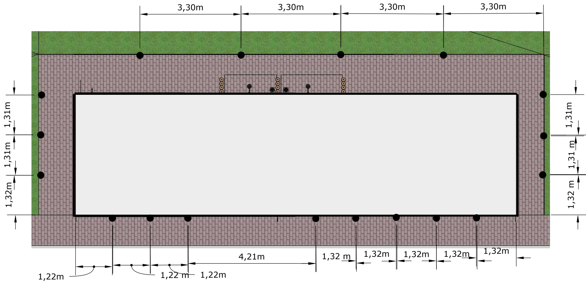
PLANTA BAIXA- PISO FACHADA ESC.:1___75
