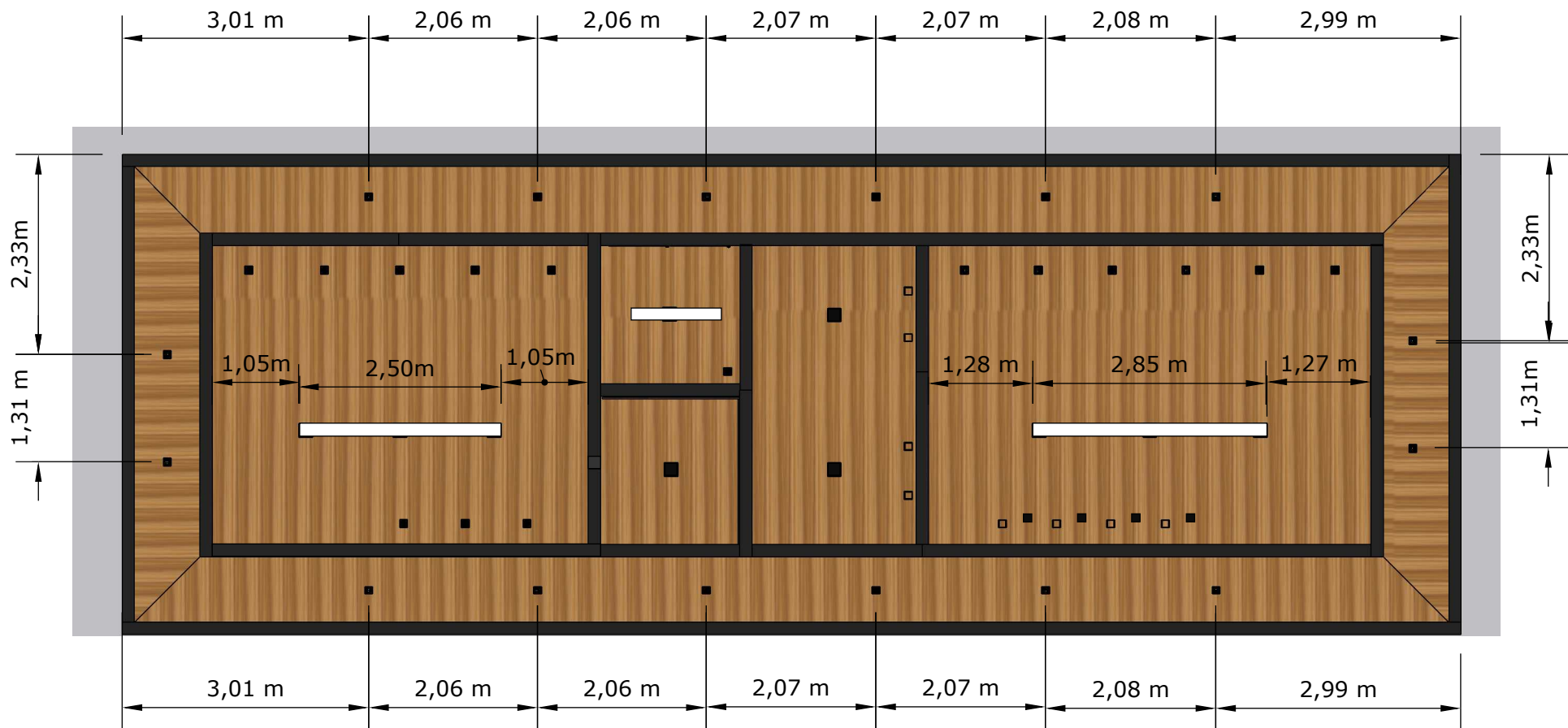
PLANTA BAIXA- FORRO INCLINADO FACHADA ESC.:1__75
